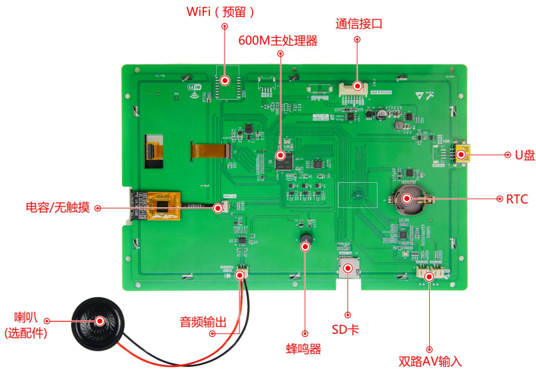
图 1-3 硬件配置图
